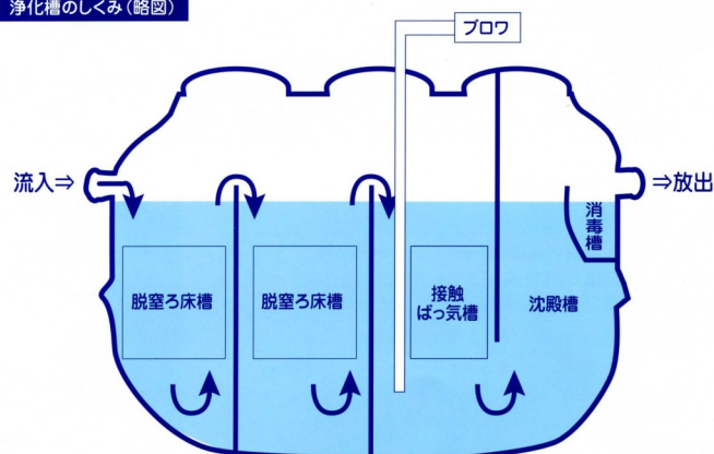
浄化槽のしくみ(略図)
