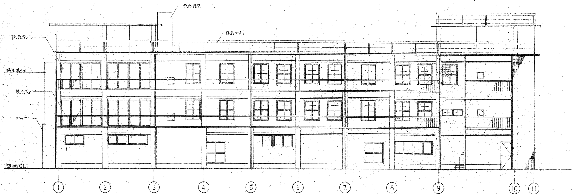
側面立面図 1:100
