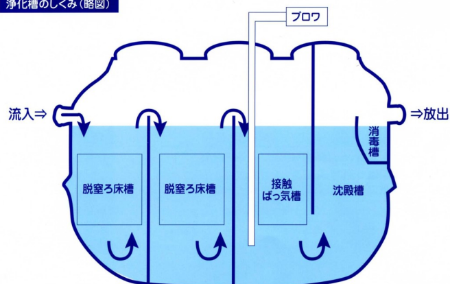
浄化槽のしくみ(略図)
